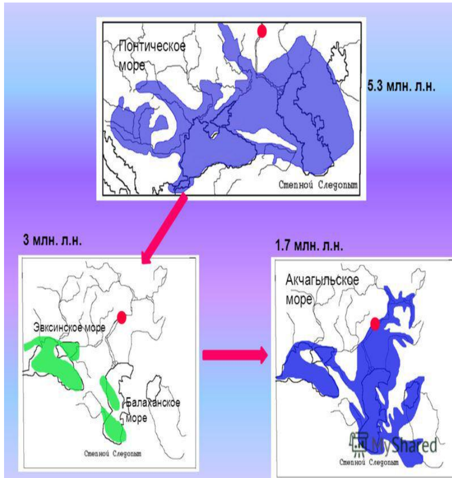
Акчагыльское море.
